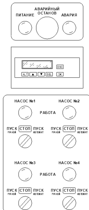
Рисунок 11. Лицевая панель ИСТОК UP на 4 насоса
