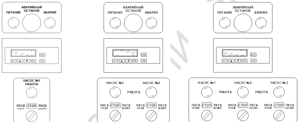
Рисунок 10. Лицевая панель ИСТОК УР на 1, 2 и 3 насоса
