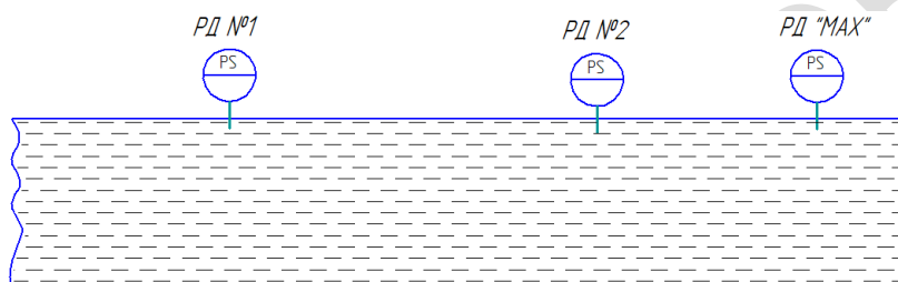
Рисунок 9. Алгоритм №8, схема расположения реле давления
